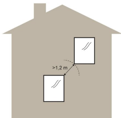
Figur 12: Exempel på lösning där fönster placeras mer än 1,2 m från underliggande fönster som ger minst samma säkerhet som det allmänna rådet. Illustration: Boverket/Altefur Development.
