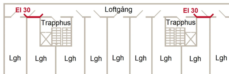
Figur 21: Då loftgång utgör enda utrymningsväg och där utformning är sådan att utrymning enbart kan ske i en riktning krävs brandteknisk avskiljning EI 30 mot de brandceller som utrymmande måste passera för att nå närmsta trapphus. Illustration: Fabian Ardin/Boverket.
