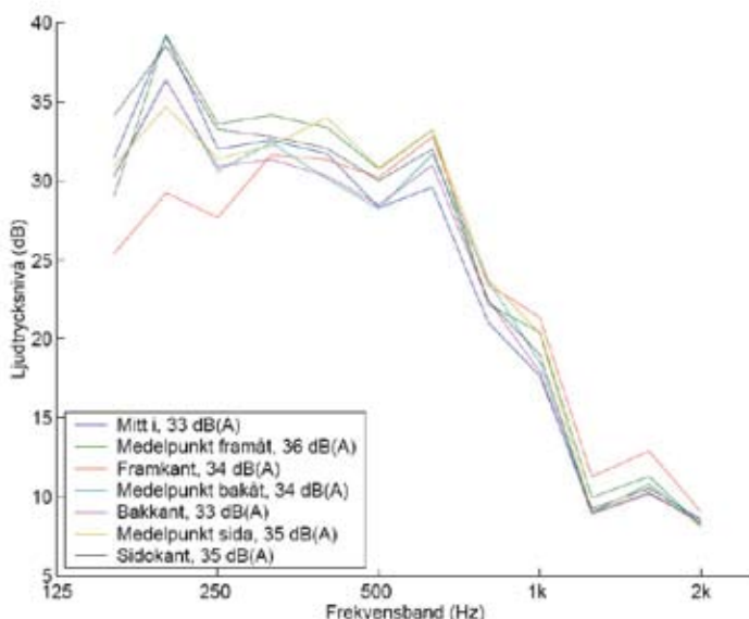
Figur 7.1 Ljudnivåer från vattentömning i WC, från 1 m höjd över vattenspegeln.
