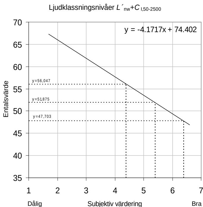
Figur 4.3 Beräknade lämpliga klassgränser med hänsyn till det standardiserade måttet, L'_{n,w} + C_{1,50-2500} efter Hagberg 17 .
