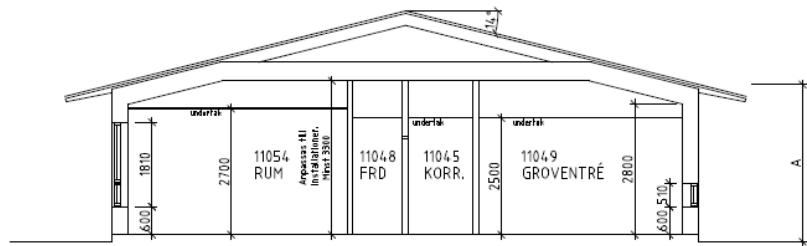
SEKTION A-A
