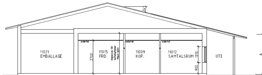
SEKTION B-B
