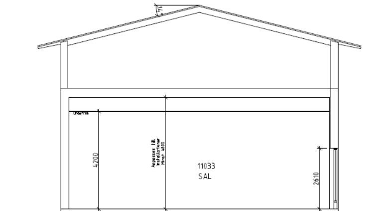
SEKTION C-C
