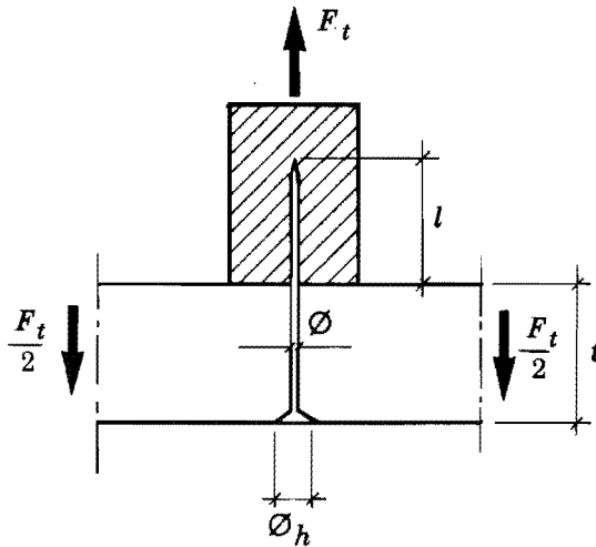
Utdragsbelastad spik.
