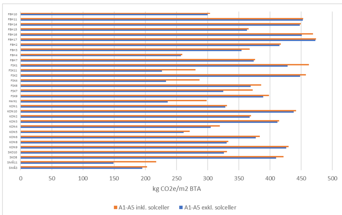
Figur 50. Jämförelse mellan klimatpåverkan modul A1-A5 inklusive respektive exklusive solcellernas klimatpåverkan för de av studiens byggnader som har solceller. Systemgräns enligt förslag på klimatdeklaration 2027.
