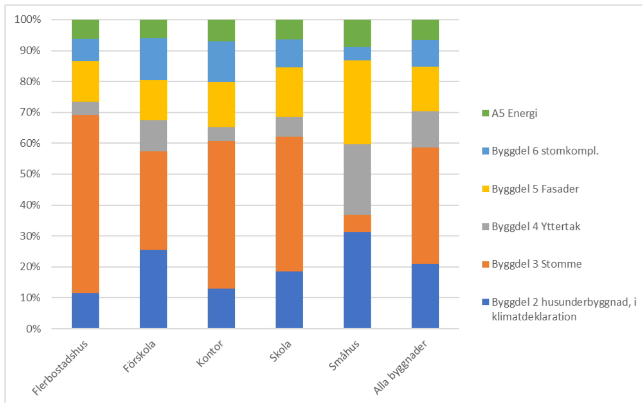
Figur 61. Andel av klimatpåverkan (A1-A5) utifrån byggdel för de olika byggnadstyperna samt för alla byggnader. Klimatpåverkan beräknad med klimatförbättrade produktval för betong, konstruktionsstål och aluminium. Systemgräns enligt klimatdeklaration 2022 . n(Småhus)=11, n(Flerbostadshus)=19, n(Förskolor)=14, n(Skolor)=10, n(Kontor)=11, , n(Alla byggnader )=68.
