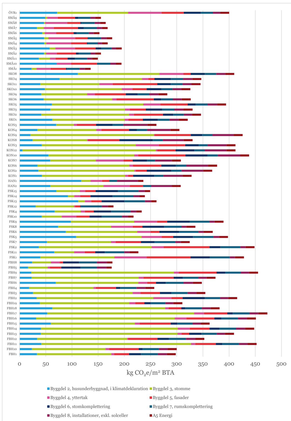
Klimatpåverkan A1-A5 Bygghälsor och A5 Energi. Utökad systemgräns för bygghälsor enligt förslag klimatdeklaration 2027 [kg CO 2 e/m 2 BTA].
