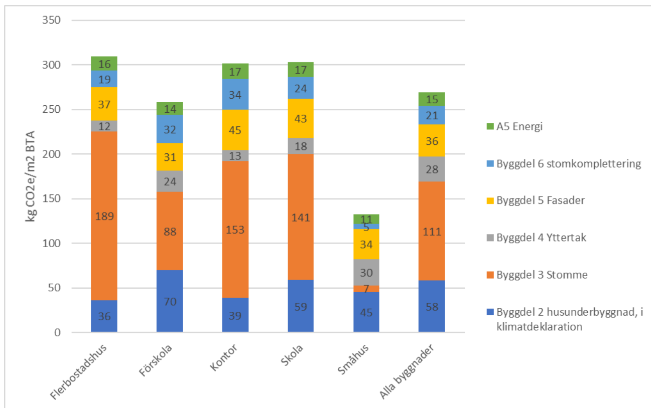
Figur 36. Medelvärde klimatpåverkan modul A1-A5. Byggdela enligt klimatdeklaration 2022 (Byggdela summerat A1-A3, A4 och A5 Spill). Kg CO2e/m2 BTA. n(Småhus)=11, n(Flerbostadshus)=19, n(Förskolor)=14, n(Skolor)=10, n(Kontor)=11, n(Alla byggnader )=68
