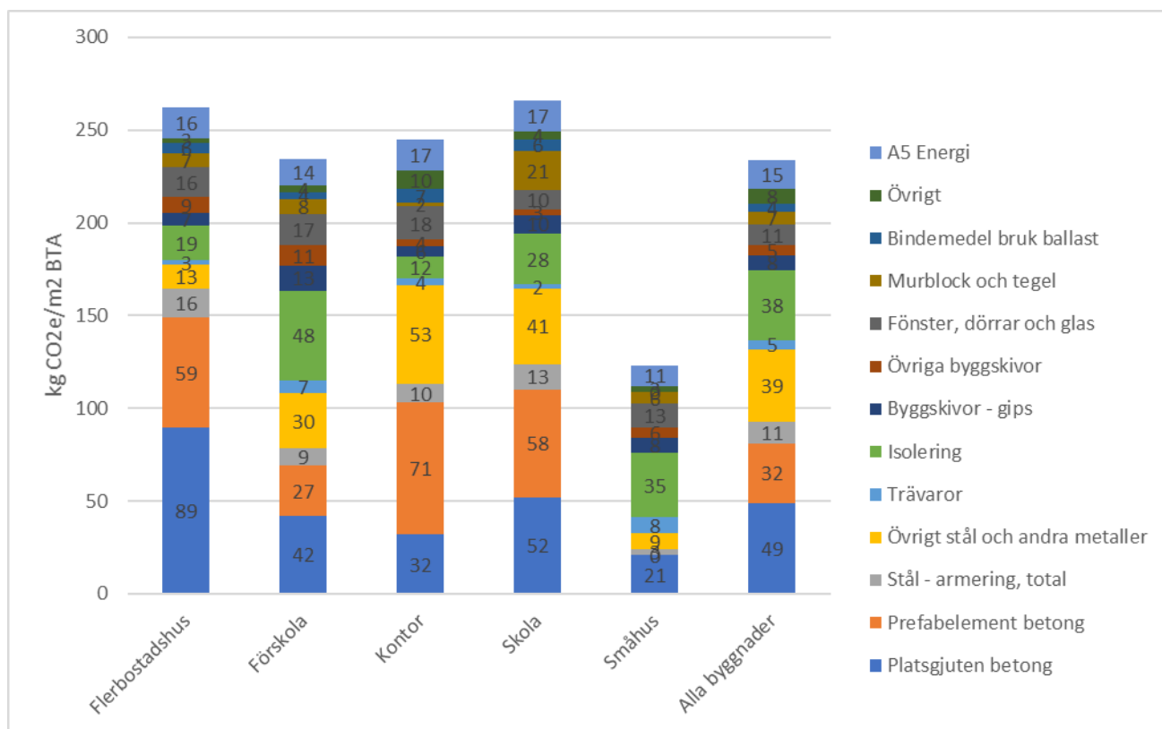
Figur 66. Fördelning av klimatpåverkan (A1-A5) utifrån produkttyp för de olika byggnadstyperna samt för alla byggnader (medelvärde). Klimatpåverkan beräknad med klimatförbättrade produktval för betong, konstruktionsstål och aluminium. Systemgräns enligt klimatdeklaration 2022 . Kg CO 2 e/m 2 BTA. n(Småhus)=11, n(Flerbostadshus)=19, n(Förskolor)=14, n(Skolor)=10, n(Kontor)=11, n(Alla byggnader)=68.
