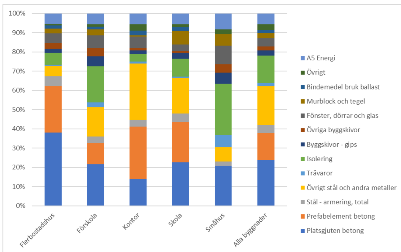
Figur 39. Andel av medelvärde klimatpåverkan modul A1-A5 indelat efter produkttyper . Inkluderade byggdelen enligt klimatdeklaration 2022 (A1-A3, A4 och A5 Spill inkluderat i produkttyper). Andel i procent. n(Småhus)=11, n(Flerbostadshus)=19, n(Förskolor)=14, n(Skolor)=10, n(Kontor)=11, , n(Alla byggnader )=68
