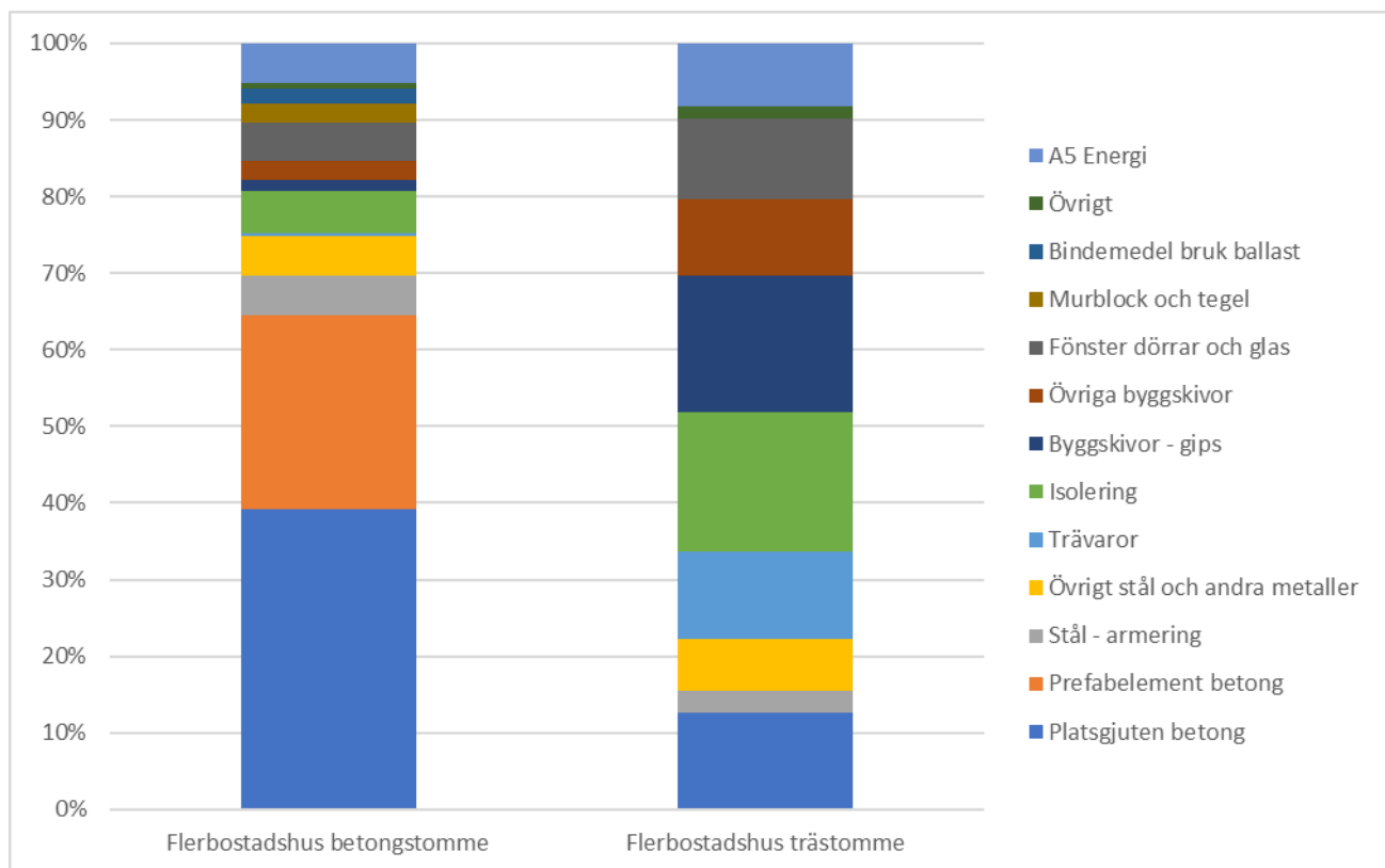
Figur 41. Medelvärde för andel av klimatpåverkan från olika produkttyper . Flerbostadshus uppdelat på olika stomtyper. A1-A5 med systemgräns 2022. n(betongstomme)=17, n(trästomme)=2
