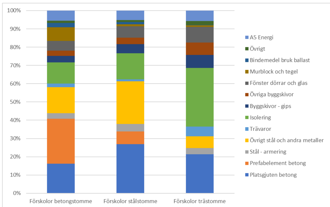
Figur 42. Medelvärde för andel av klimatpåverkan från olika produkttyper . Förskolor uppdelat på olika stomtyper. A1-A5 med systemgräns 2022. n(betongstomme)=4, n(stålstomme)=4, n(trästomme)=6
