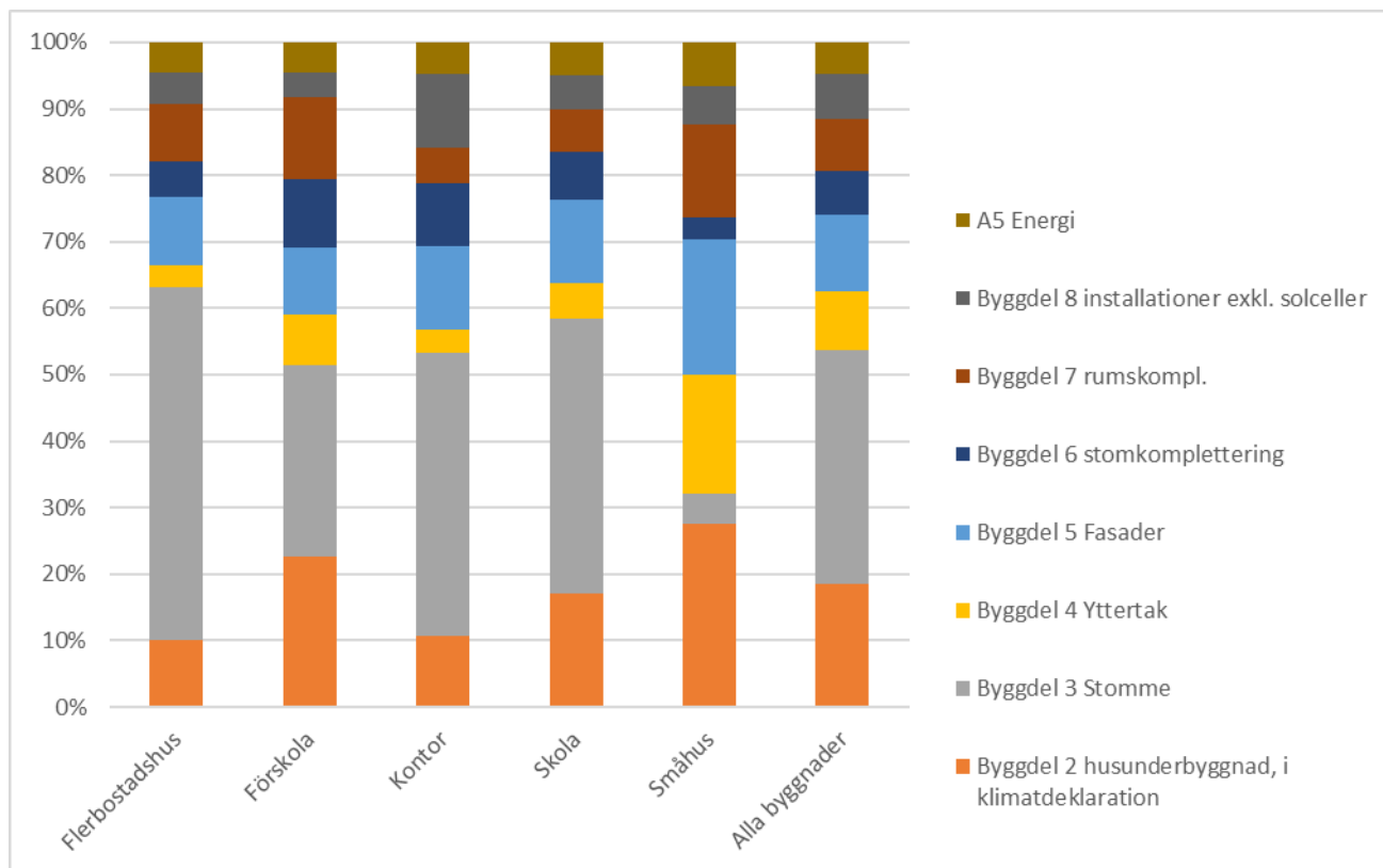
Figur 37. Andel av medelvärde klimatpåverkan modul A1-A5. Byggdela enligt förslag klimatdeklaration 2027 (Byggdela summerat A1-A3, A4 och A5 Spill). Andel i procent. n(Småhus)=11, n(Flerbostadshus)=19, n(Förskolor)=14, n(Skolor)=10, n(Kontor)=11, n(Alla byggnader )=68
