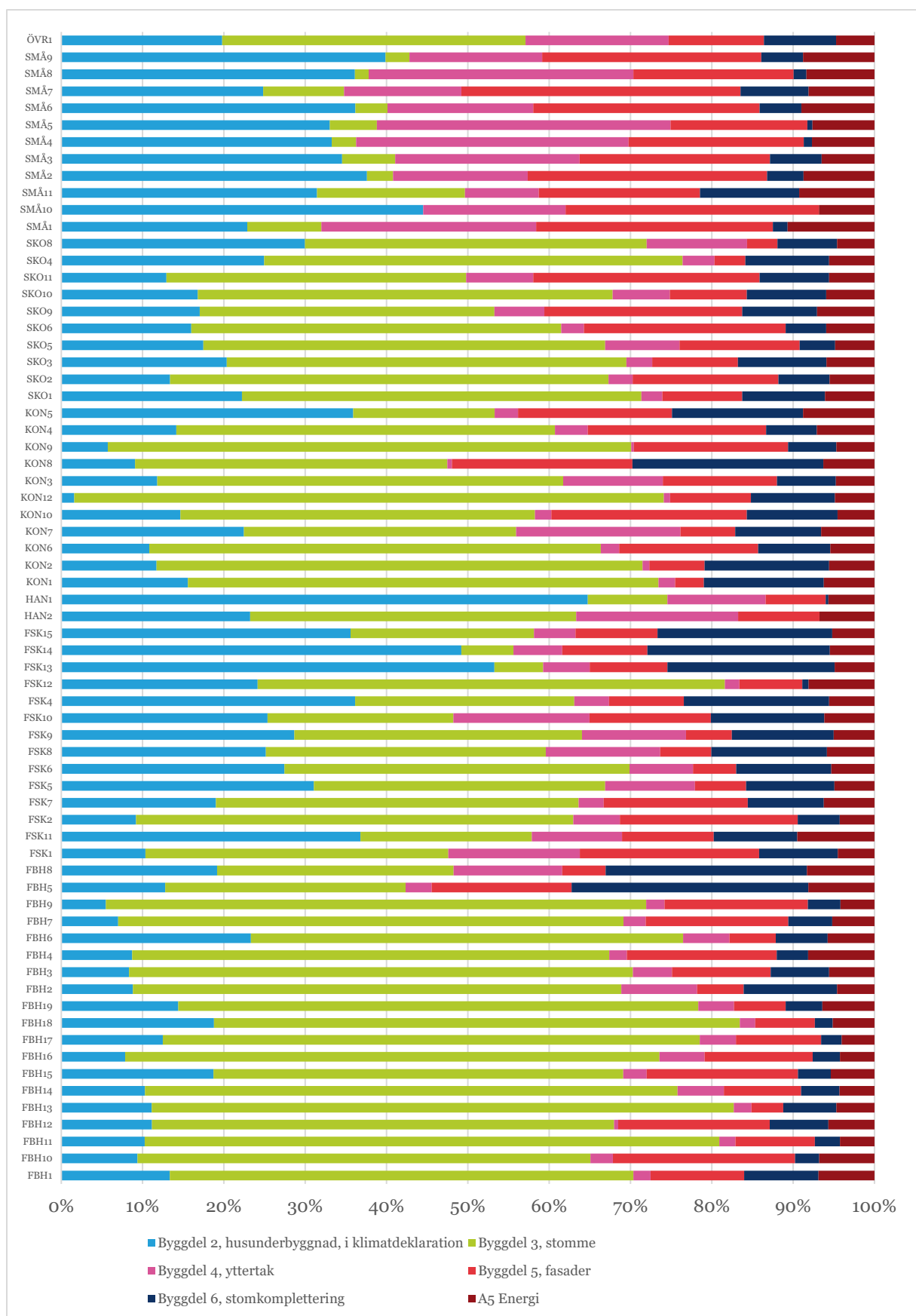
Relativ klimatpåverkan A1-A5 Bygghetar och A5 Energi. Systemgräns enligt klimatdeklaration 2022 [kg CO 2 e/m 2 BTA].
