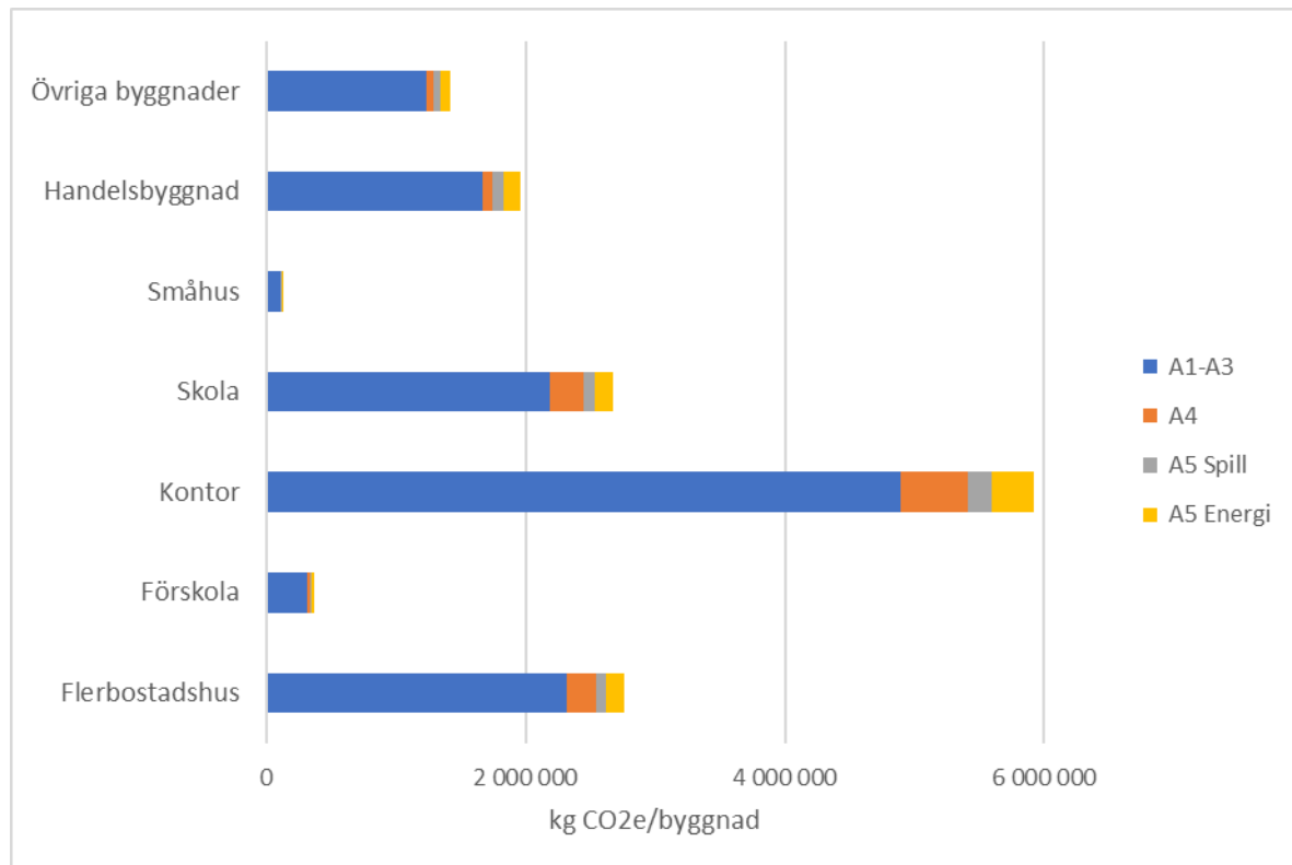
Figur 32. Total klimatpåverkan per byggnad, medelvärde per byggnadstyp. Byggheterna enligt 2022 års systemgräns. n(Småhus)=11, n(Flerbostadshus)=19, n(Förskolor)=14, n(Skolor)=10, n(Kontor)=11, n(Handelsbyggnader)=2, n(Övriga byggnader)=1
