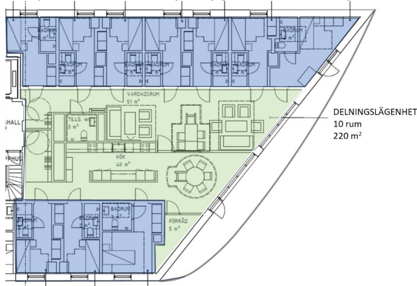
(figur 2) Delningsbostad om 10 boendeenheter
