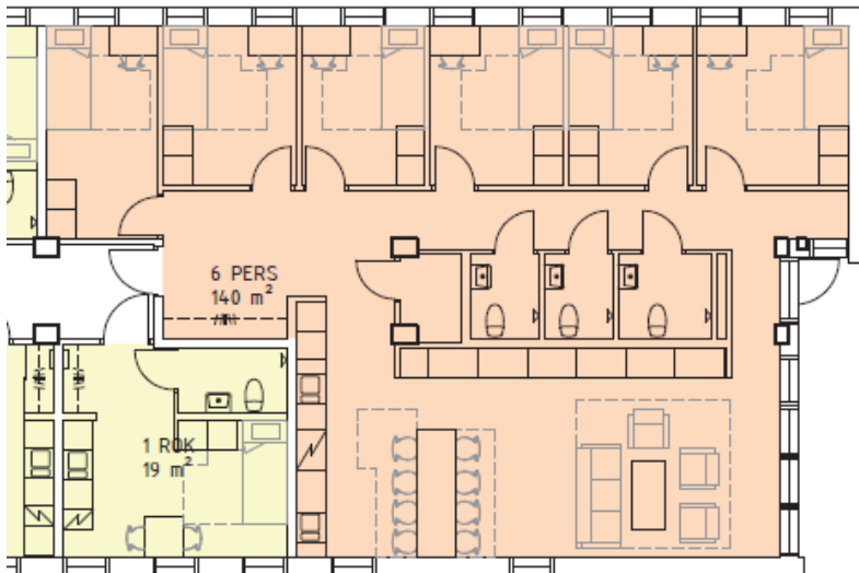
(figur 3) - Delningsbostad om 6 boendeenheter
